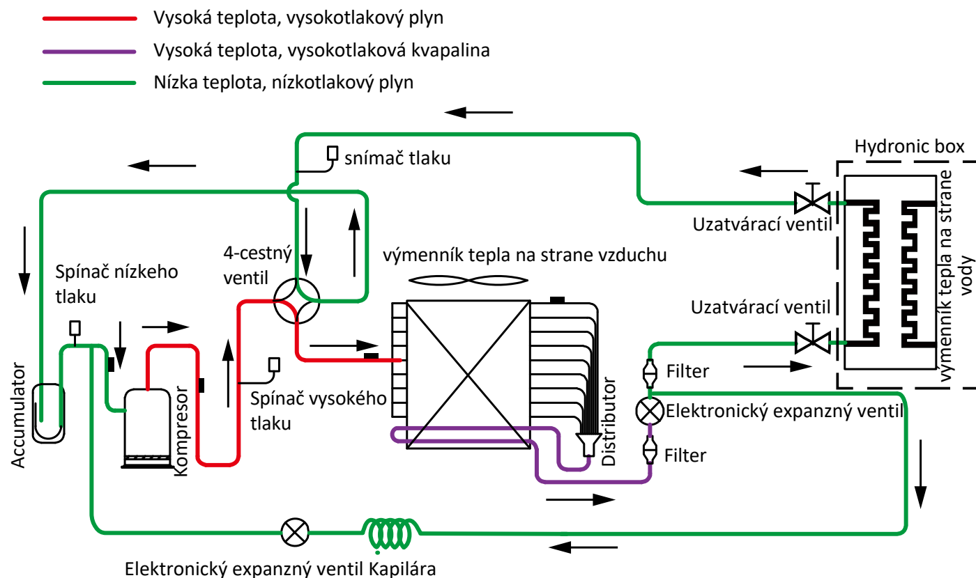
Obrázok 2-3.2: Tok chladiva počas prevádzky chladenia a rozmrazovania
