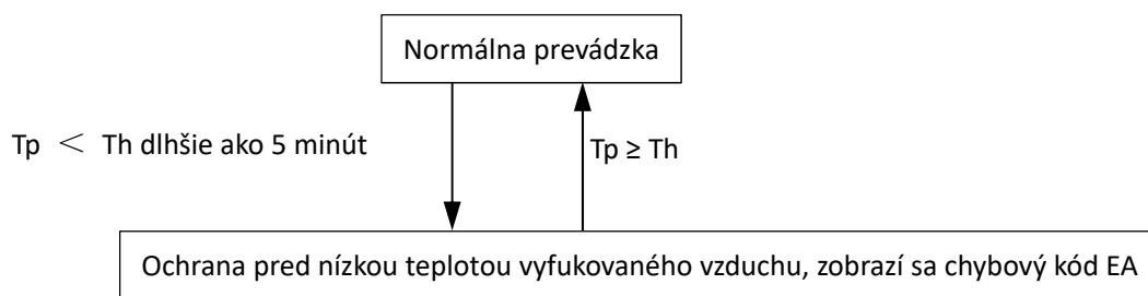
Obrázok 3-5.4: Riadenie ochrany pred nízkou teplotou chladivo
