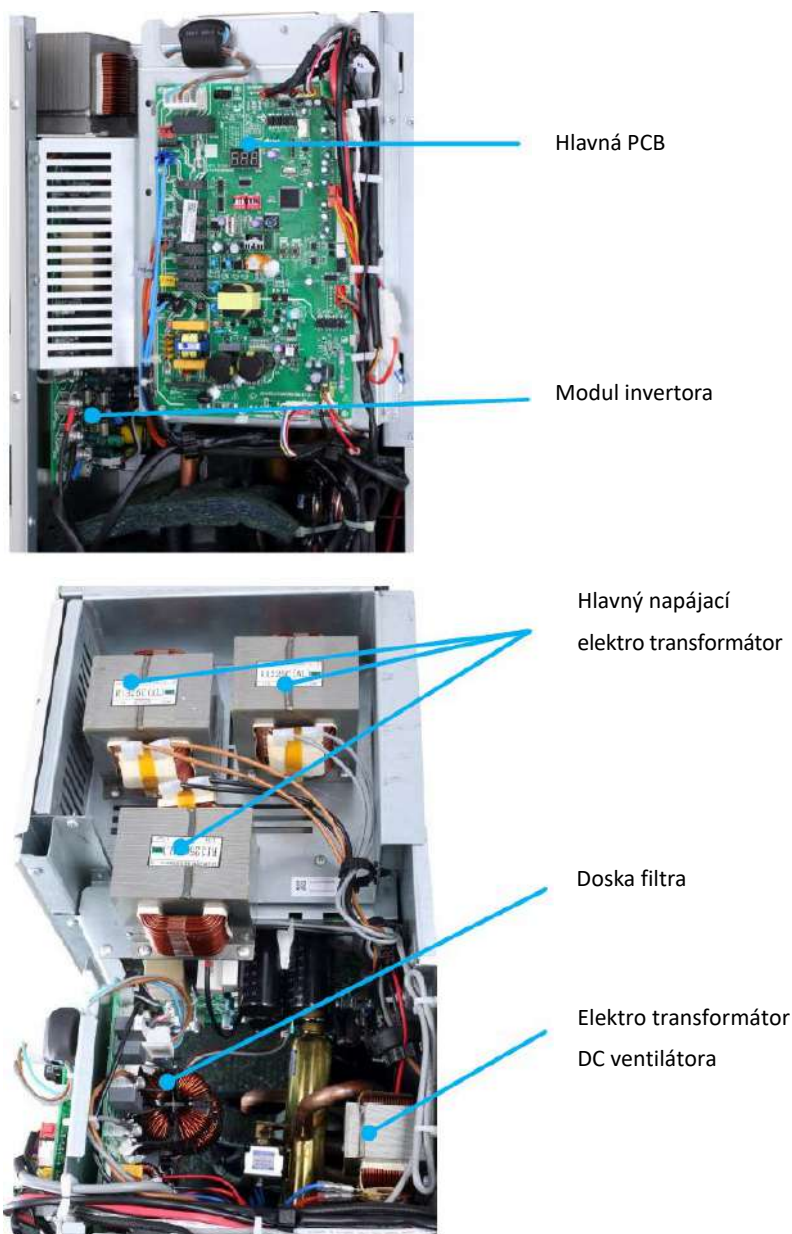
Obrázok 4-1.4: HOP12(14,16)WODU3, elektrický rozvádzač
