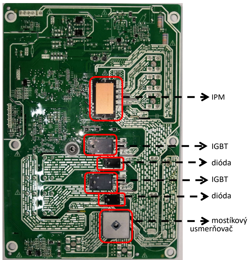
Obrázok 4-5.2: Výmena modulu invertora
