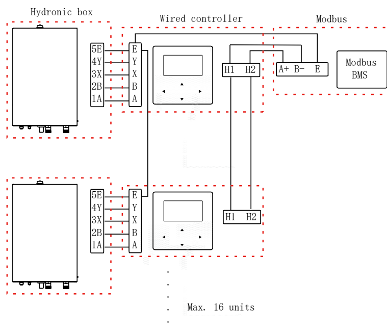
Obrázok 4-2.11: Zapojenie
