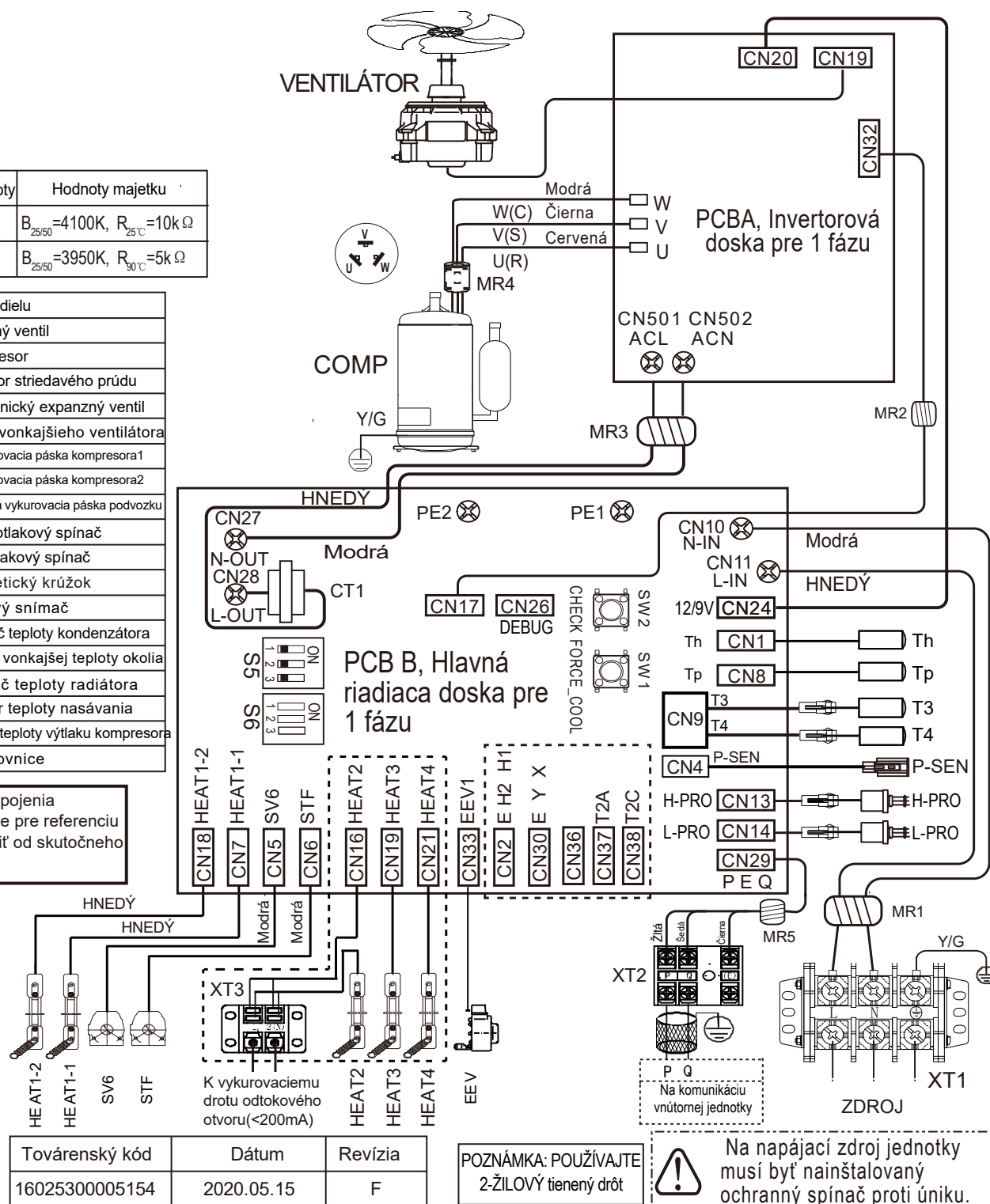
Obrázok 4-3.1: HOP4(6,8,10)WODU schéma zapojenia
