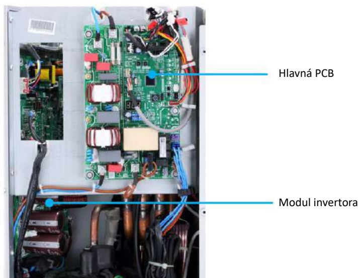
Obrázok 4-1.3: HOP12(14,16)WODU, elektrický rozvádzač
