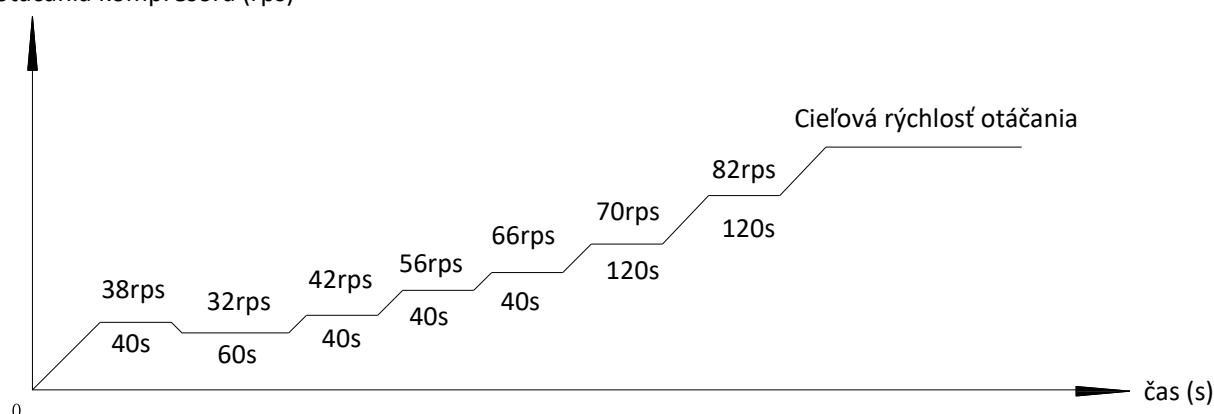
Obrázok 3-3.1: HOP4(6)WODU, program na spustenie kompresora 1 , keď je teplota vonkajšieho prostredia vyššia ako 3 °C
