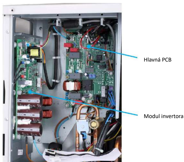
Obrázok 4-1.2: HOP8(10)WODU, elektrický rozvádzač
