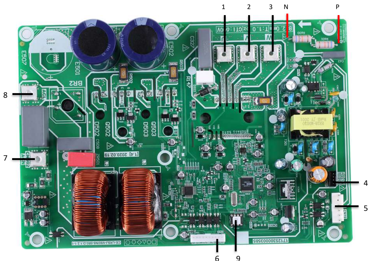
Obrázok 4-2.5 HOP4(6,8,10)WODU, modul invertora pre vonkajšiu jednotku Pre model s výkonom 4/6kW
