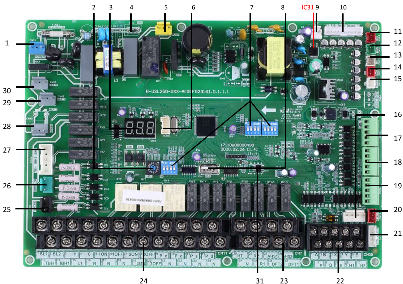
Obrázok 4-2.1: Hlavná PCB hydronického boxu HOP60(100,160)WIDU(3)
