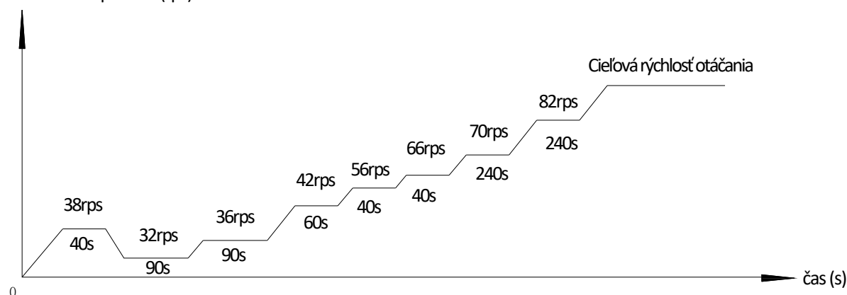
Obrázok 3-3.2: HOP4(6)WODU, program na spustenie kompresora 1 , keď je teplota vonkajšieho prostredia 3 °C alebo menej
