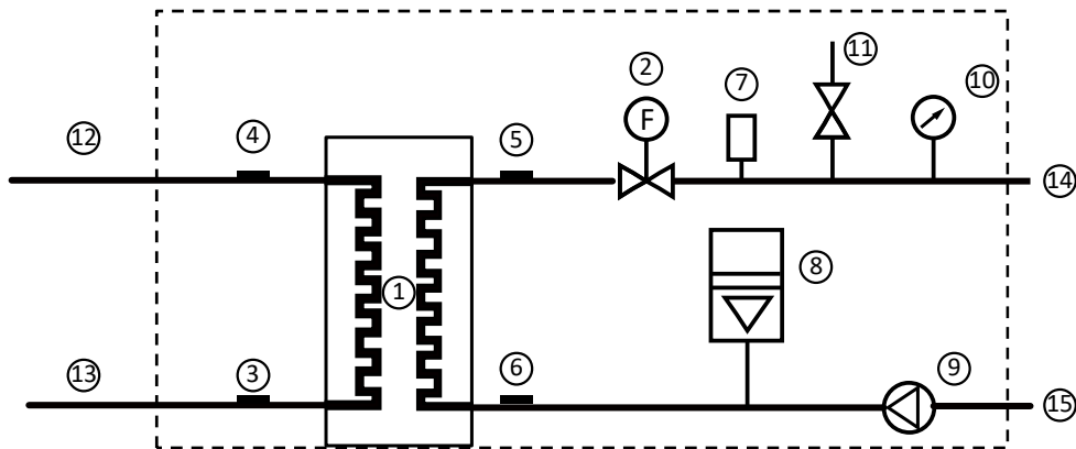
Obrázok 2-2.2: Schéma potrubných vedení hydronického boxu
