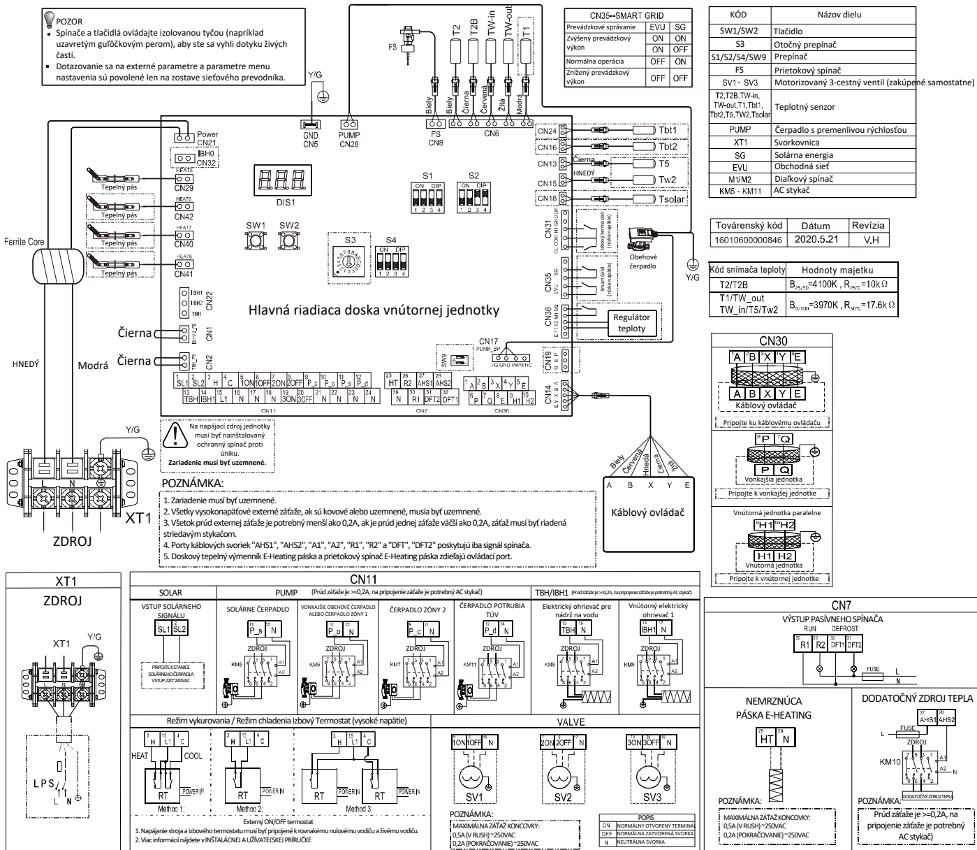
Obrázok 4-3.2 HOP60(100,160)WIDU(3) schéma zapojenia
