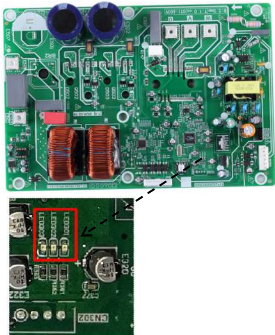
Obrázok 4-5.1: Umiestnenie LED na module invertora
