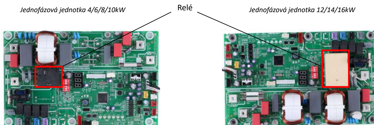
Obrázok 4-5.4: Umiestnenie relé na hlavnej PCB chladiaceho systému
