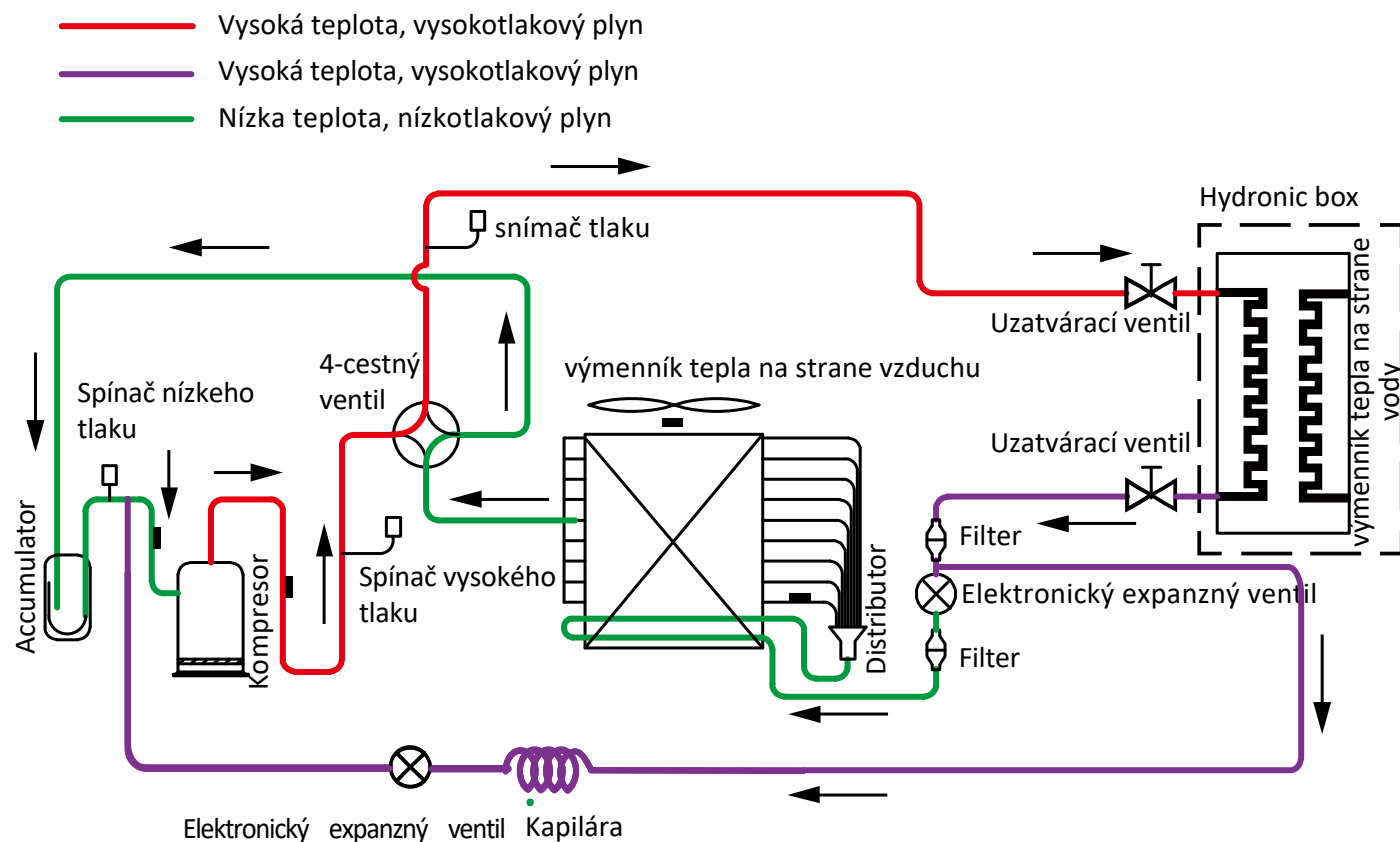
Obrázok 2-3.1: Tok chladiva počas prevádzky ohrevu alebo úžitkovej teplej vody
