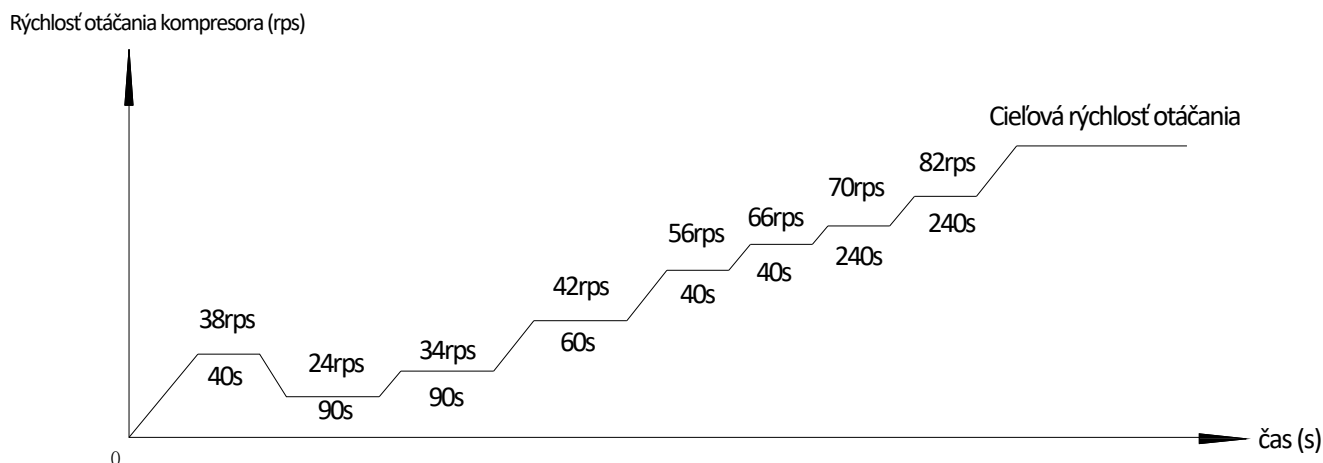
Obrázok 3-3.6: HOP12(14,16)WODU(3), program na spustenie kompresora1, keď je teplota vonkajšieho prostredia 3 °C alebo menej
