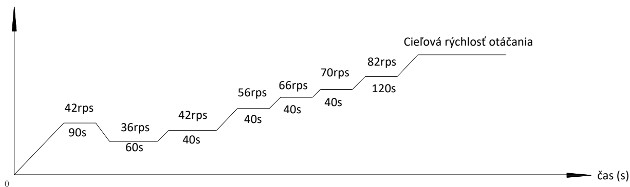
Obrázok 3-3.3: HOP8(10)WODU, program na spustenie kompresora 1 , keď je teplota vonkajšieho prostredia vyššia ako 11 °C
