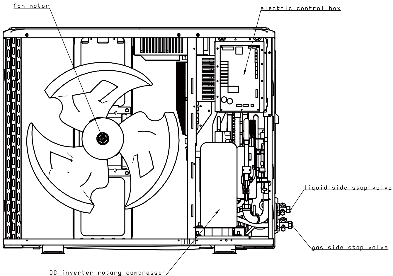
Obrázok 2-1.8: HOP12(14,16)WODU3, pohľad spredu
