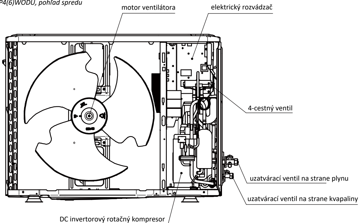
Obrázok 2-1.2: HOP4(6)WODU, pohľad spredu
