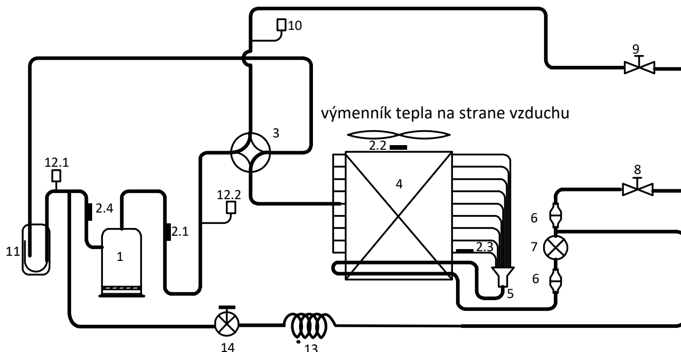
Obrázok 2-2.1: Schéma potrubných vedení vonkajšej jednotky
