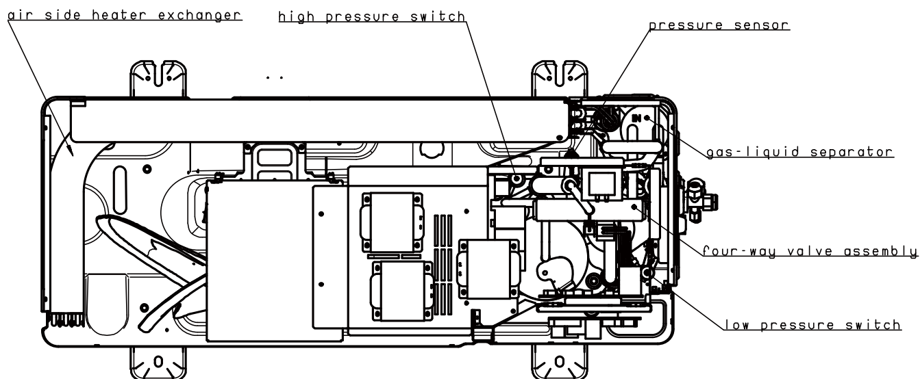
Obrázok 2-1.7: HOP12(14,16)WODU3, pohľad zvrchu
