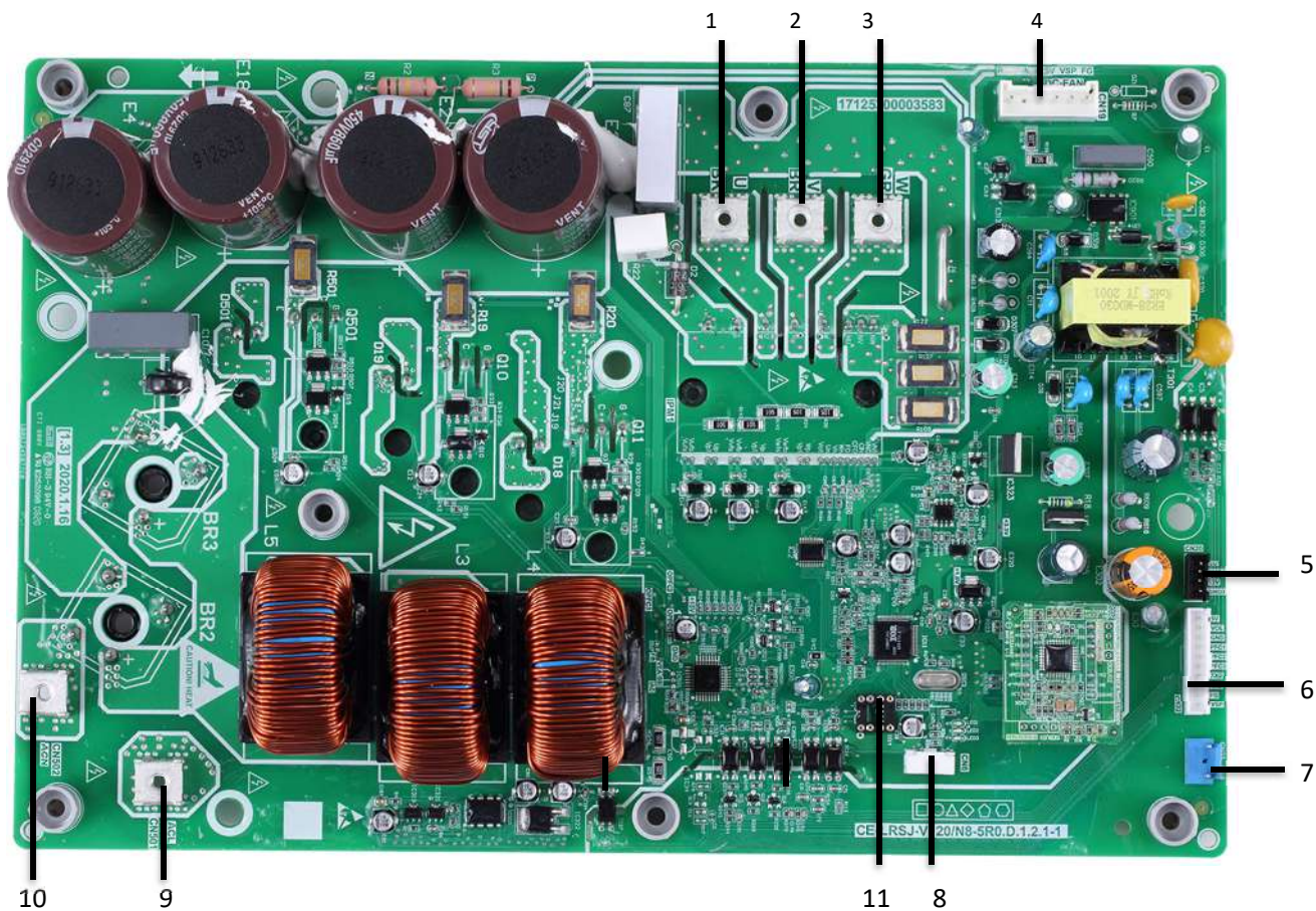
Obrázok 4-2.6: HOP12(14,16)WODU, modul invertora pre vonkajšiu jednotku
