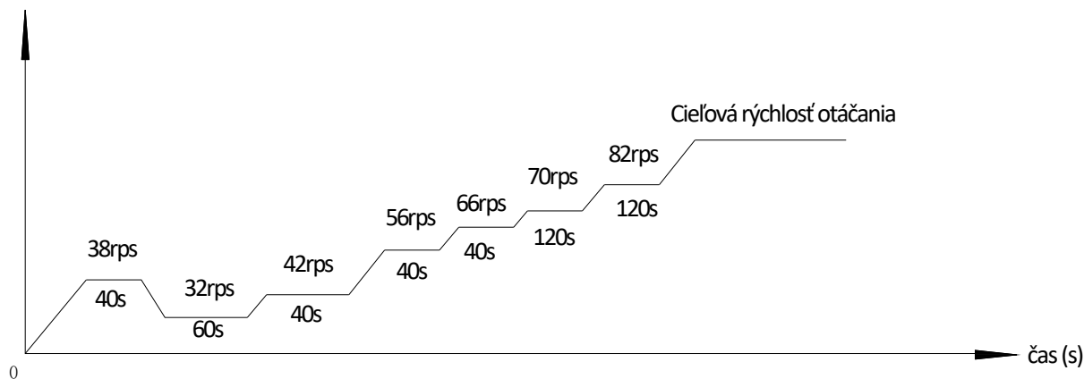
Obrázok 3-3.5: HOP12(14,16)WODU(3), program na spustenie kompresora 1 , keď je teplota vonkajšieho prostredia vyššia ako 3 °C
