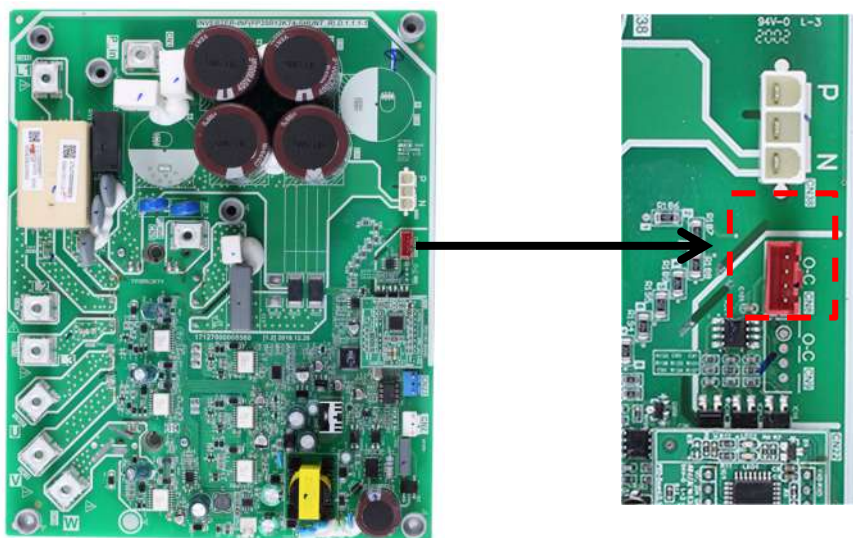
Obrázok 4-5.8: Zapojenie portu pre modul invertora
