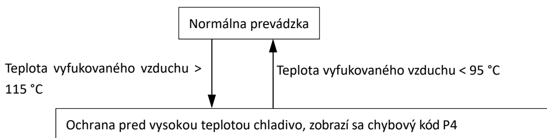
Obrázok 3-5.3: Riadenie ochrany pred vysokou teplotou chladivo
