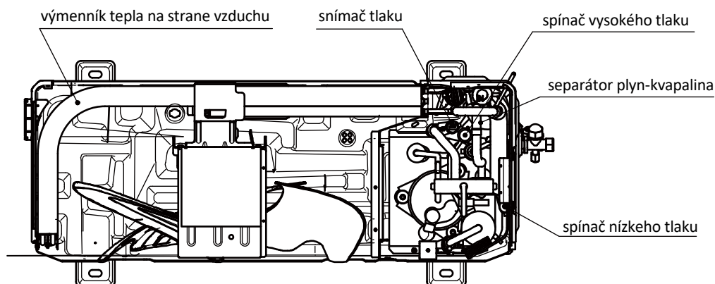
Obrázok 2-1.1: HOP4(6)WODU, pohľad zvrchu
