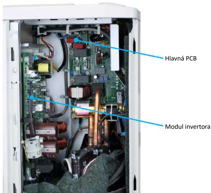
Obrázok 4-1.1: HOP4(6)WODU, elektrický rozvádzač
