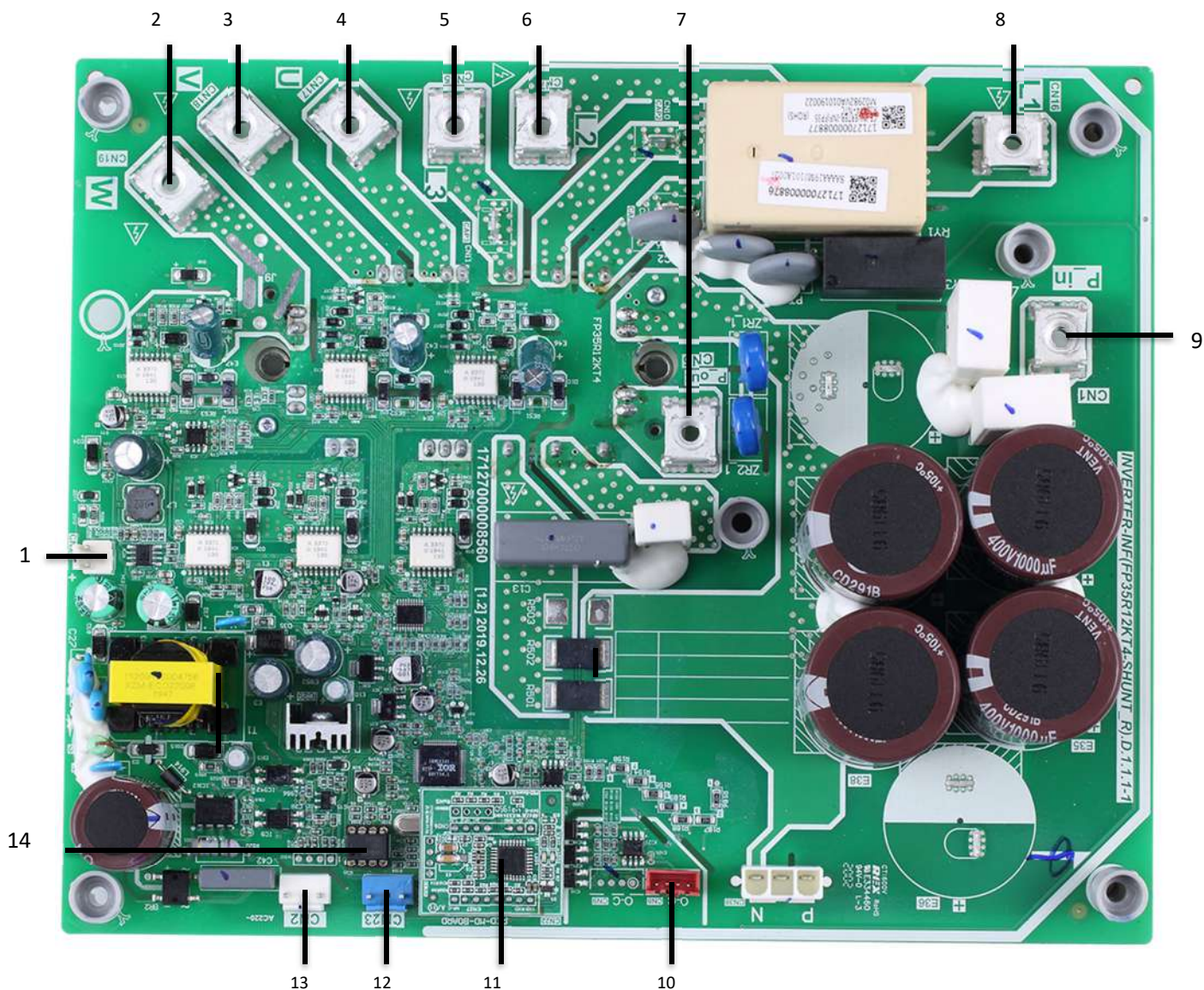
Obrázok 4-2.7: HOP12(14,16)WODU3, modul invertora pre vonkajšiu jednotku
