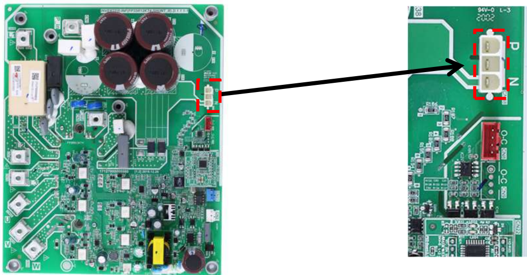
Obrázok 4-5.9: Napätie na svorkách P, N
