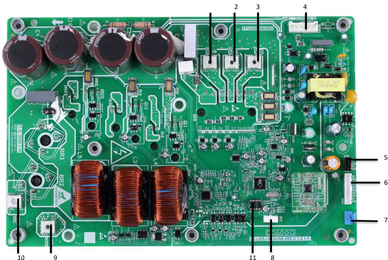
Obrázok 4-2.6: HOP12(14,16)WODU, modul invertora pre vonkajšiu jednotku
