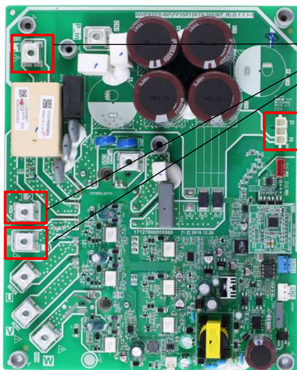
Obrázok 4-5.11: Mostíkový usmerňovač
