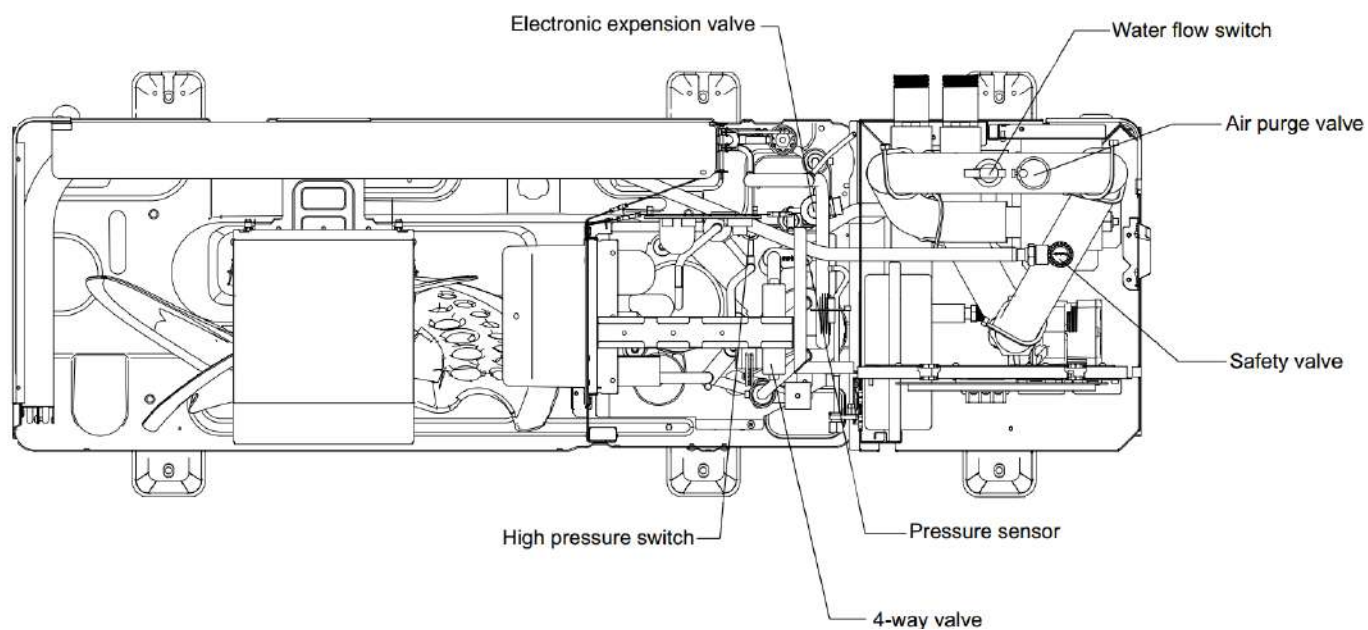
Obrázok 2-1.2: HOP8(10)WMONO, pohľad spredu
