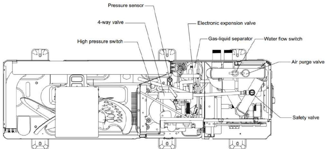
Obrázok 2-1.4: HOP12(14,16)WMONO, pohľad zvrchu
