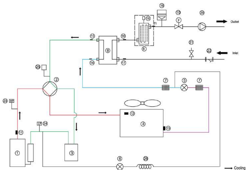
Obrázok 2-2.2: Režim chladenia
