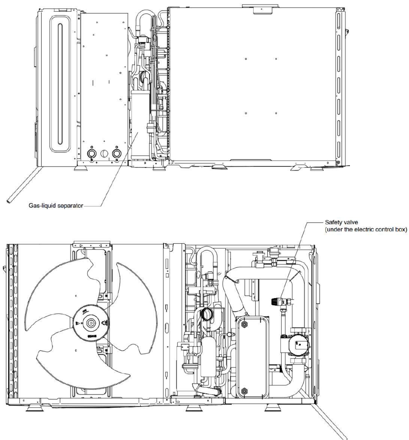
Obrázok 2-1.3: HOP4(6)WMONO
