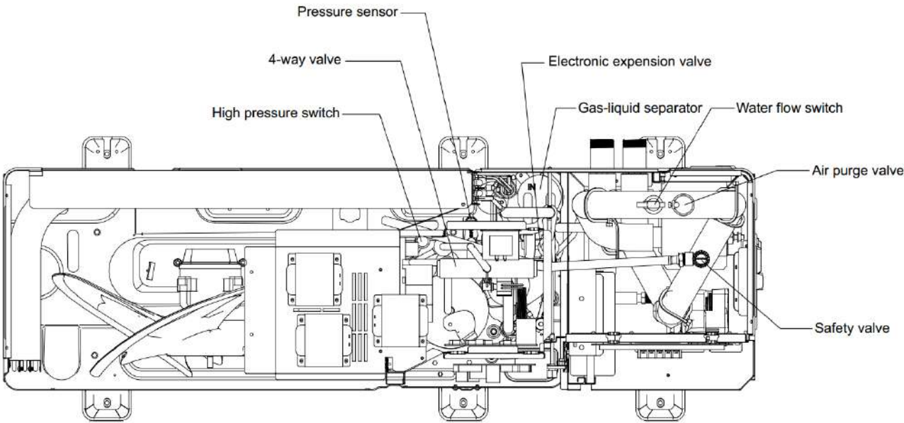
Obrázok 2-1.5: HOP12(14,16)WMONO, HOP12(14,16)WMONO3, pohľad spredu
