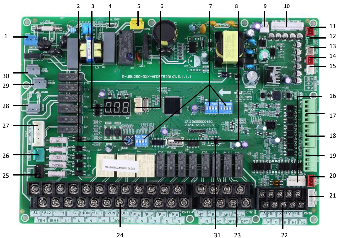
Obrázok 4-2.1: Hlavná PCB pre hydronický systém vonkajšej jednotky
