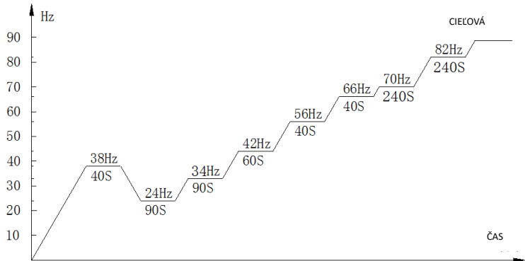
Obrázok 3-3.4: 12-16KW, program na spustenie kompresora 1 , keď je teplota okolia rovná alebo nižšia ako 3°C
