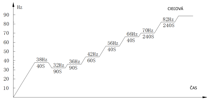
Obrázok 3-3.4: 12-16KW, program na spustenie kompresora 1 , keď je teplota okolia rovná alebo nižšia ako 3°C
