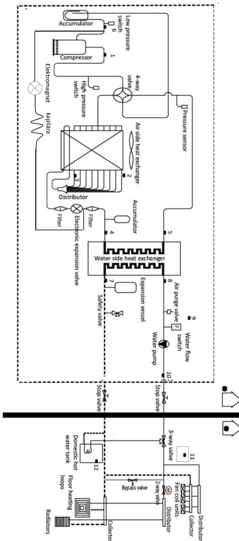
Obrázok 3-7.1: Poloha snímačov teploty v systémoch jednotiek 4~16KW
