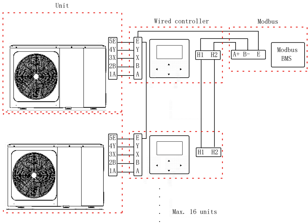
Obrázok 4-2.11: Schéma
