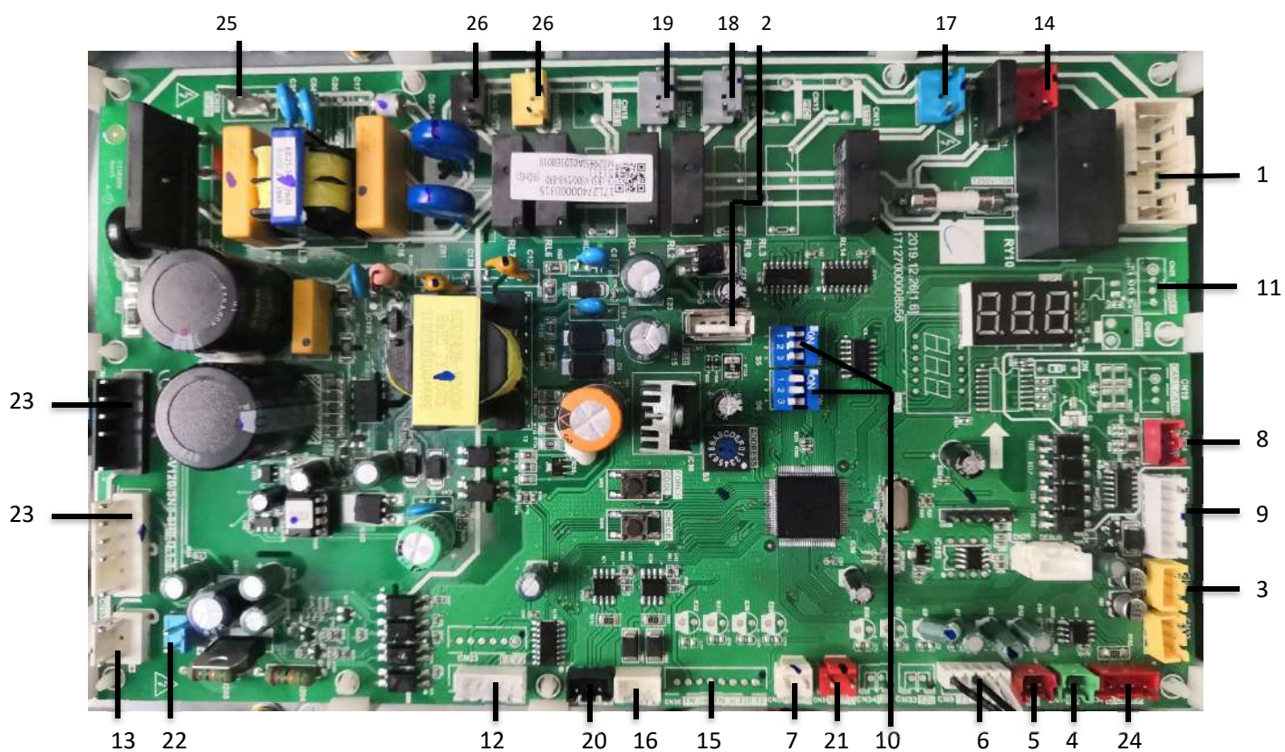
Obrázok 4-2.2: HOP18(22,26,30)WMONO3, hlavná PCB vonkajšej jednotky pre chladiaci systém
