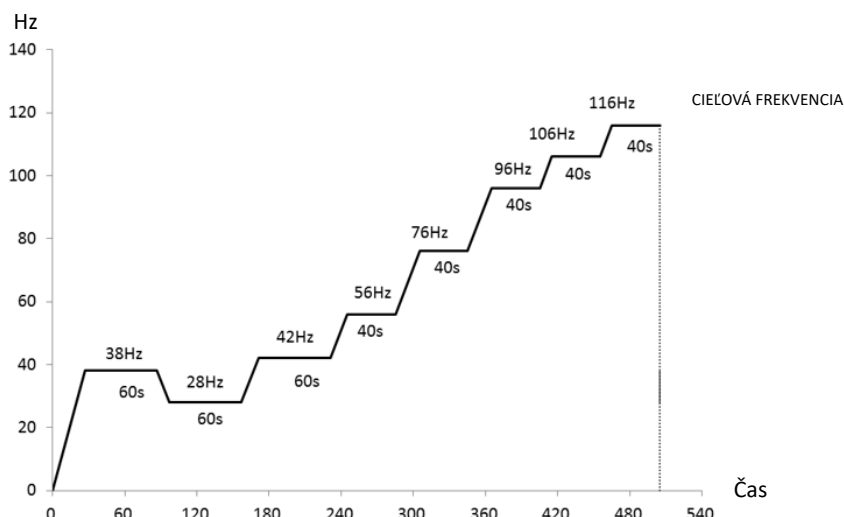
Obrázok 3-3.1 Program spúšťania kompresora 18-30 kW v režime 1
