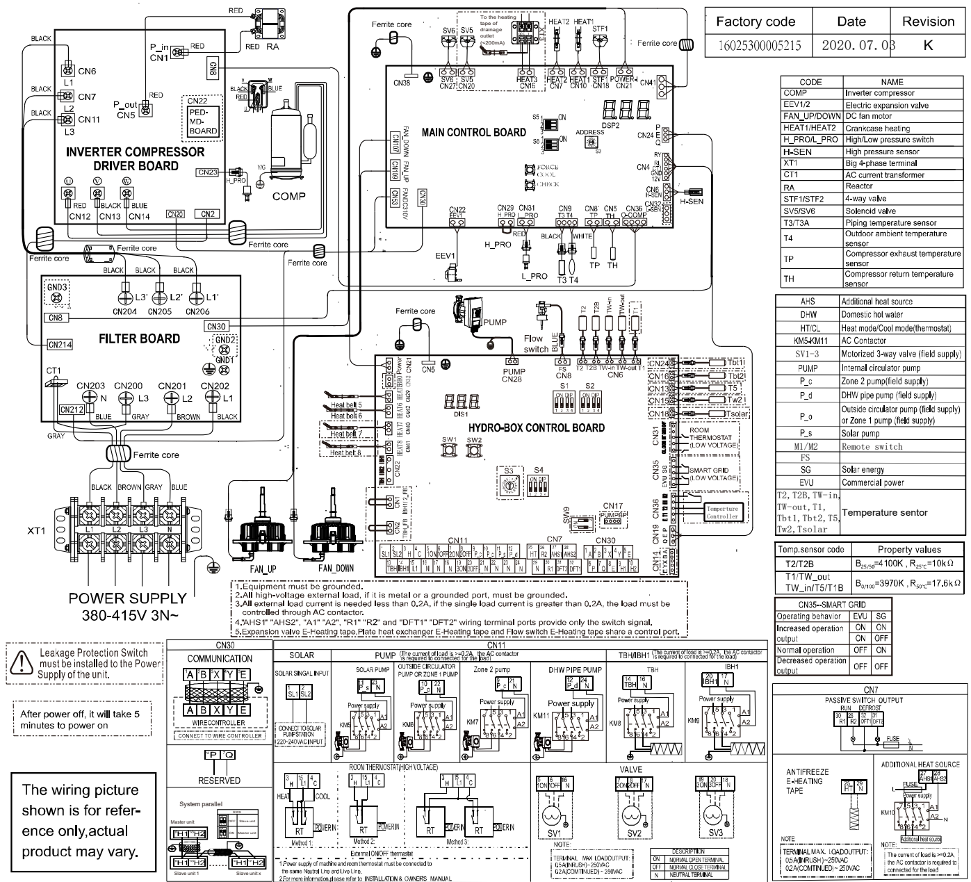
Obrázok 4-3.1: HOP18(22, 26,30)WMONO3, schéma zapojenia
