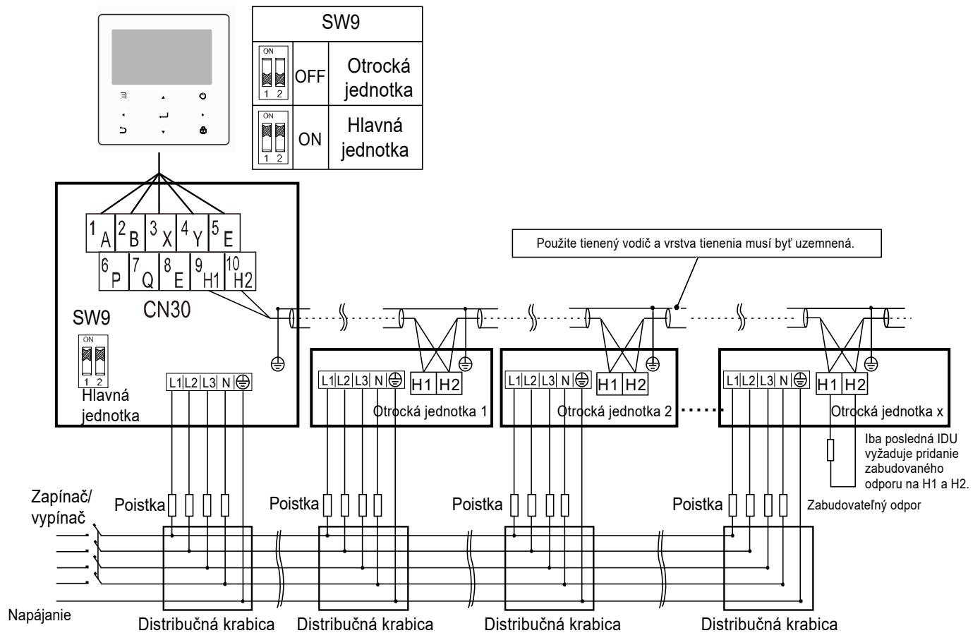
Obrázok 4-3.2: HOP18(22, 26,30)WMONO3, schéma zapojenia systému skupinového riadenia
