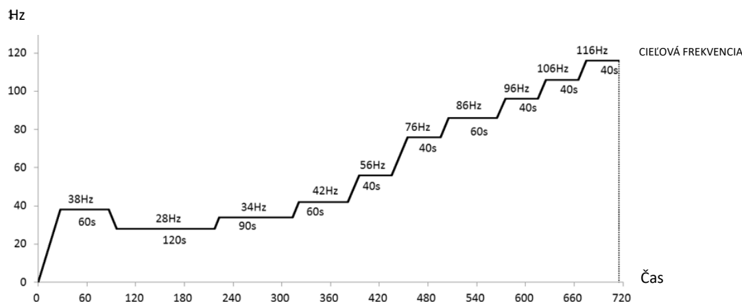
Obrázok 3-3.2 Program spúšťania kompresora 18-30 kW v režime 2
