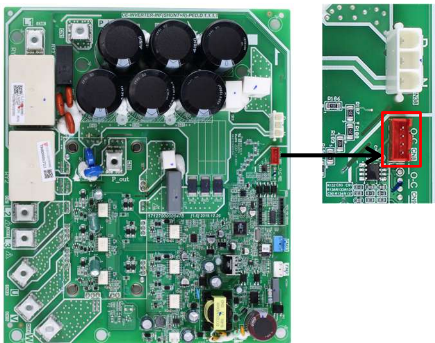
Obrázok 4-5.5: Zapojenie portu for modul invertora
