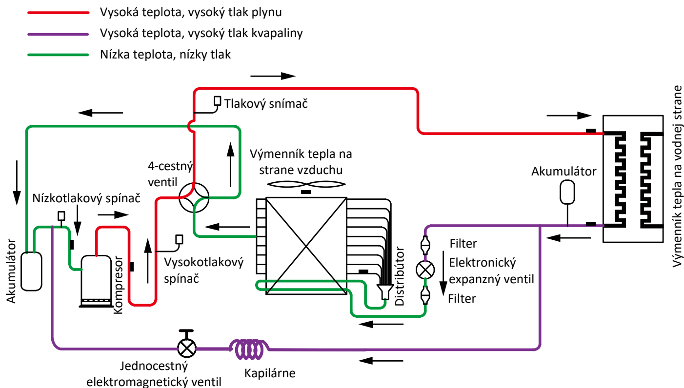
Obrázok 2-3.1: Tok chladiva počas prevádzky ohrevu alebo úžitkovej teplej vody
