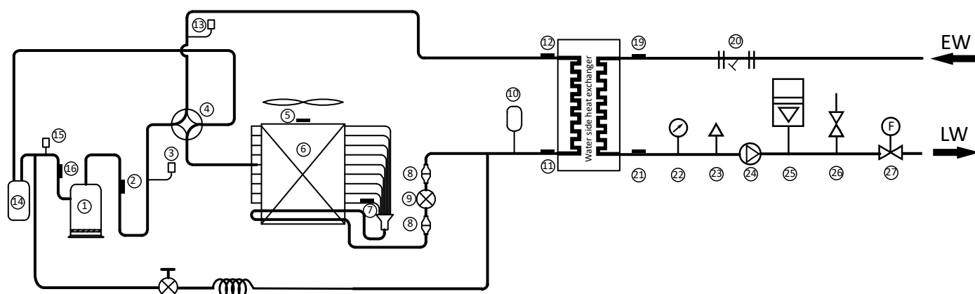
Obrázok 2-2.1: HOP18(22,26,30)WMONO3, schéma pneumatického zapojenia
