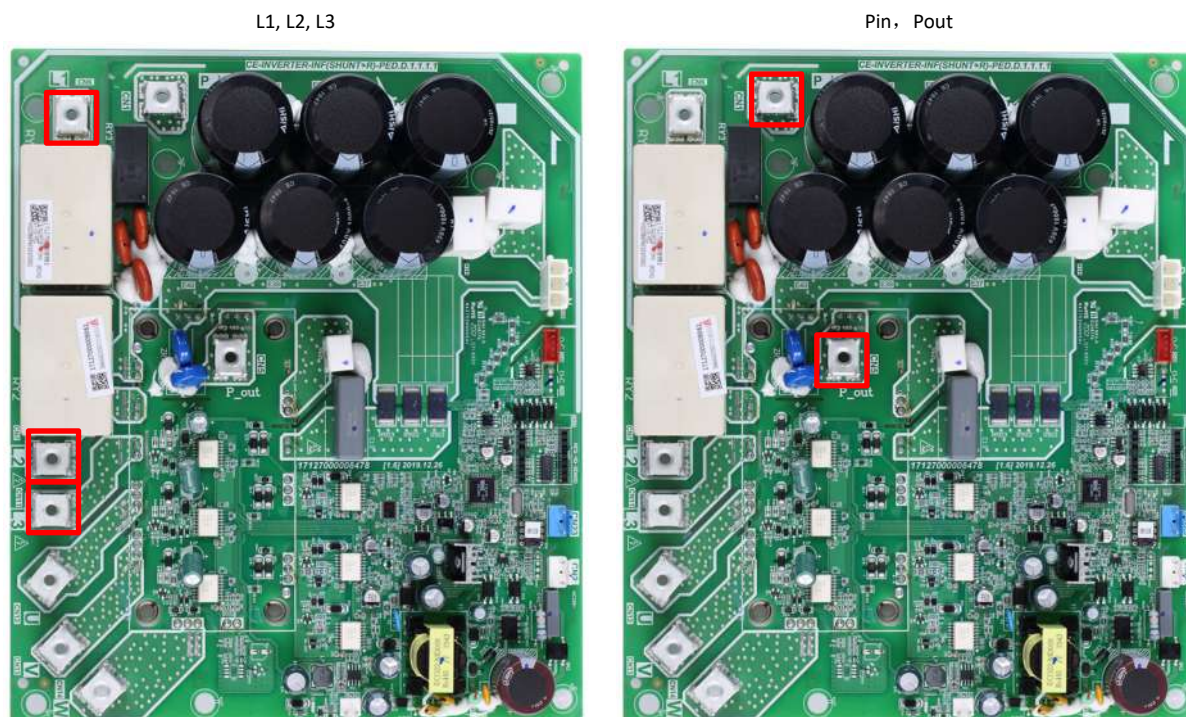
Obrázok 4-5.4: Zapojenie kábla DC zbernice (L1L2L3, PIN- POUT)
