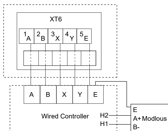
Obrázok 4-2.7: Schéma
