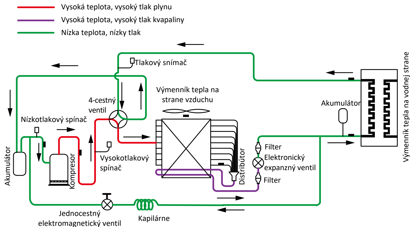
Obrázok 2-3.2: Tok chladiva počas prevádzky chladenia a rozmrazovania
