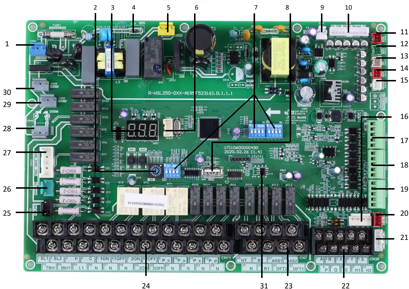
Obrázok 4-2.1: HOP18(22,26,30)WMONO3, hlavná PCB hydronického systému
