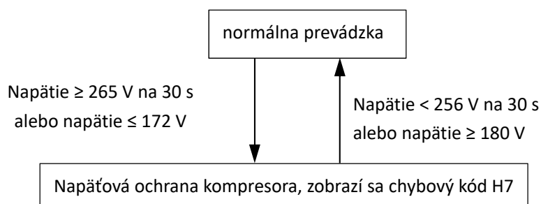
Obrázok 3-5.6: Riadenie napätovej ochrany kompresora
