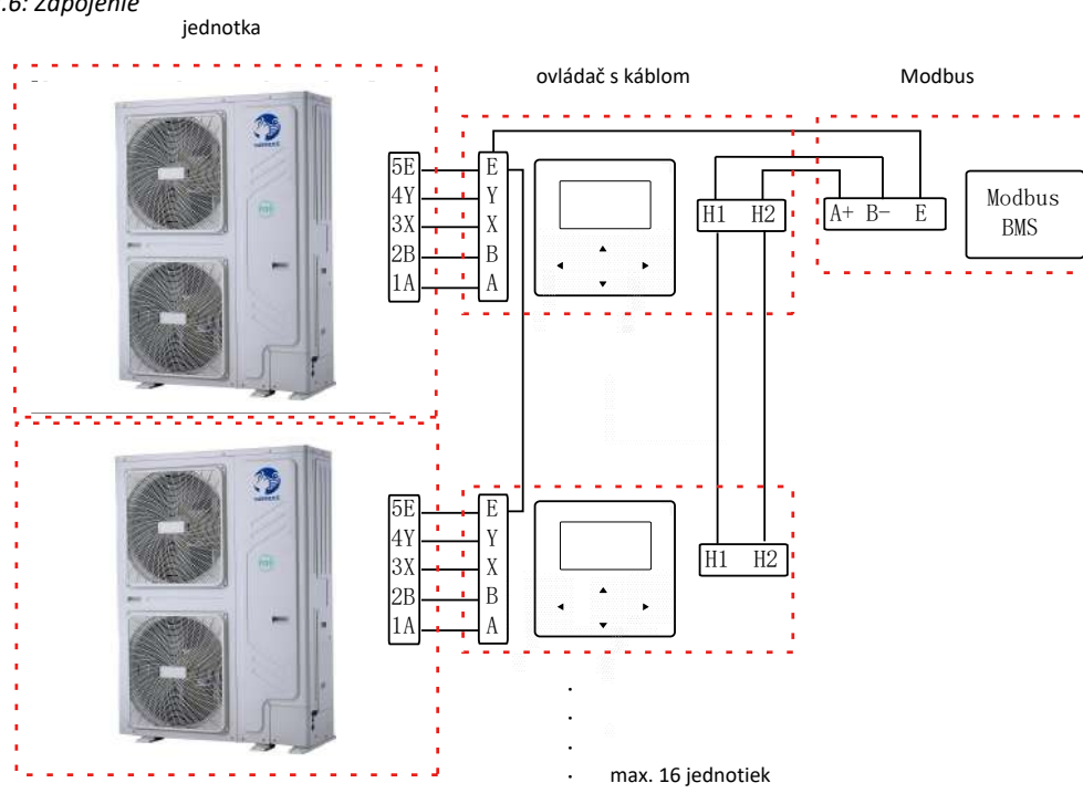
Obrázok 4-2.7: Schéma
