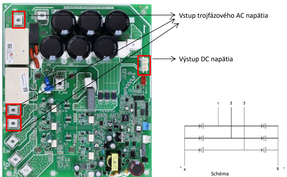
Obrázok 4-5.8: Mostíkový usmerňovač
