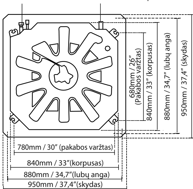
18-48K „Super-Slim“ modelių lubų skylės dydis
