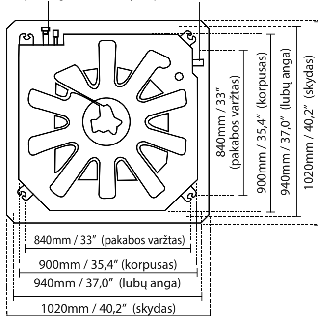
60K „Super-Slim“ modelių lubų skylės dydis
