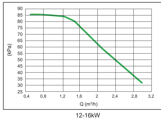
Доступное внешнее статическое давление VS Расход
