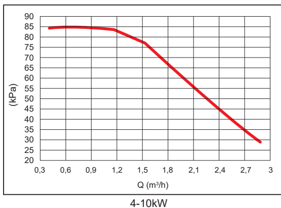
Доступное внешнее статическое давление VS Расход
