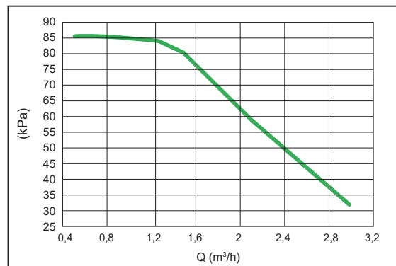
Presiune statică externă disponibilă VS Debit
