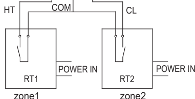
Metoda C (Controlul zonei duble)
