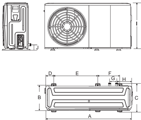
4/6 kW (Einheit: mm)
