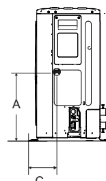
8/10/12/14/16 kW (jednotka:mm)
