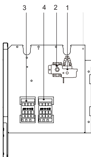
1-fázový 8-16kW se záložním ohříváčem(1-fázový 3kW) 3-fázový 12-16kW se záložním ohříváčem(1-fázový 3kW)
