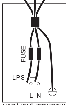
NAPÁJENÍ JEDNOTKY 1-fázový
