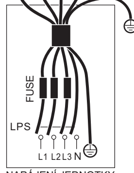
NAPÁJENÍ JEDNOTKY 3-fázový
