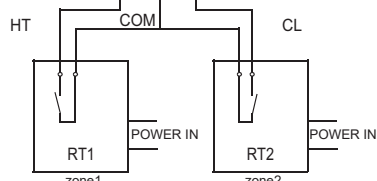
Metoda C (Dvouzónové ovládání)
