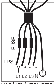
NAPÁJENÍ JEDNOTKY 3-fázový
