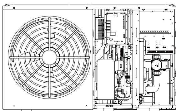
Chladicí systém
