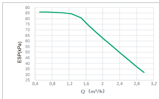
Pressione statica esterna disponibile VS Portata
