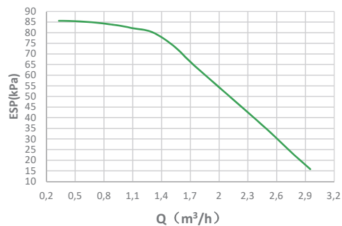
Pressione statica esterna disponibile VS Portata
