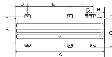
8/10/12/14/16 kW (unità: mm)
