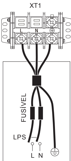
ALIMENTAÇÃO DA UNIDADE DE INTERIOR (Modelos básicos)
