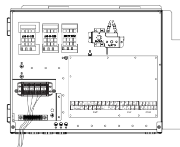
NOTRANJA ENOTA NAPAJALNIK 3-fazni 9kW rezervni grelnik po želji
